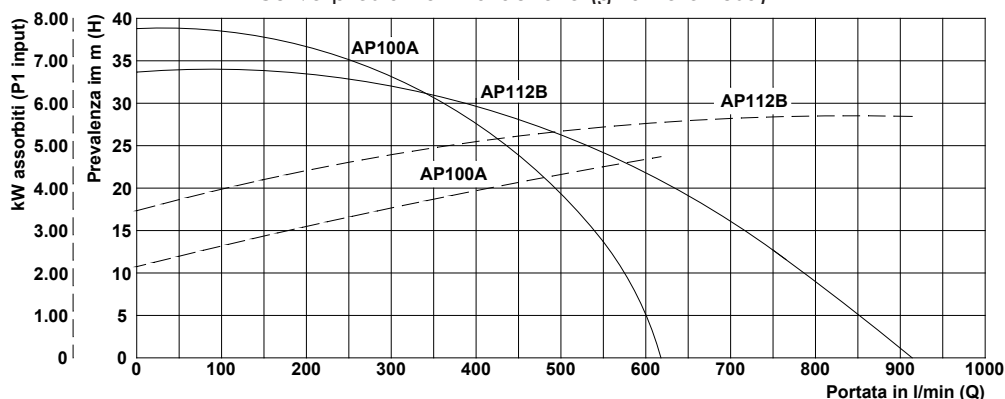
Curve prestazioni idrauliche (girante chiusa)
