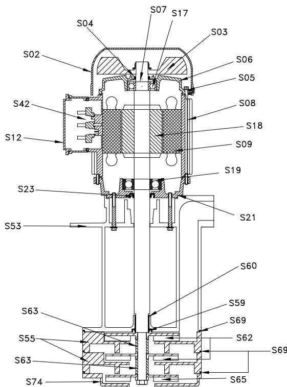
Nomenclatura parti di ricambio
