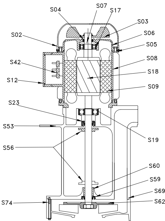
Nomenclatura parti di ricambio
