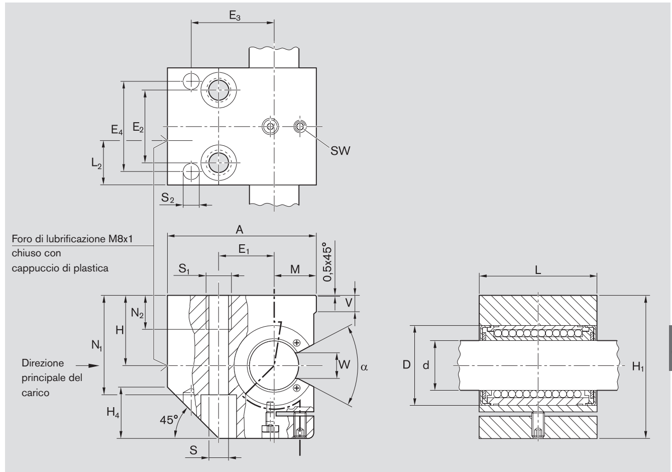
Dimensioni (mm)
