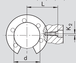
Diametri dell'albero 30, 40, 50, 60, 80
