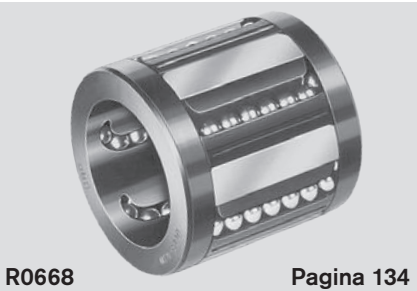
R0668 Pagina 134 Manicotto a sfere Segmentario
