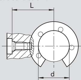
Diametro dell'albero 20
