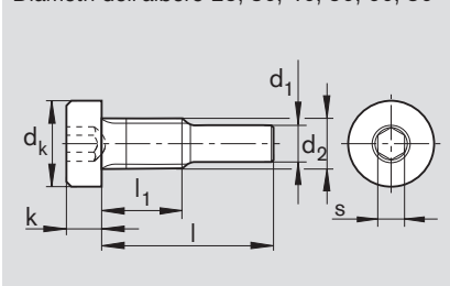
Diametri dell'albero 25, 30, 40, 50, 60, 80
