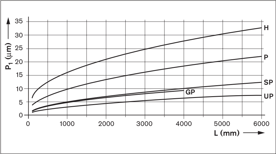
Legenda della figura P_1 = Errore di parallelismo ( \mu\text{m} ) L = Lunghezza rotaia (mm)
